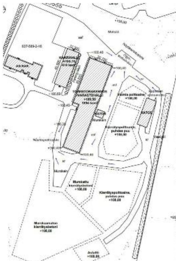
Kuva 2. Hulevesien johtaminen.
