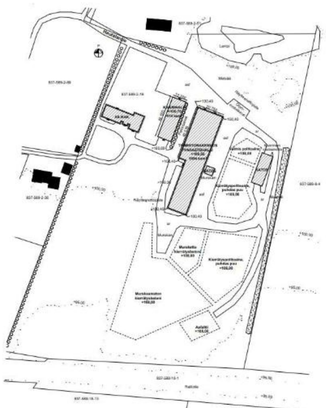
Kuva 1. Asemapiirros.
